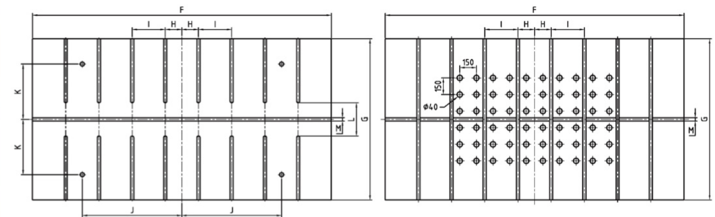
平板尺寸 Bolster Dimension
