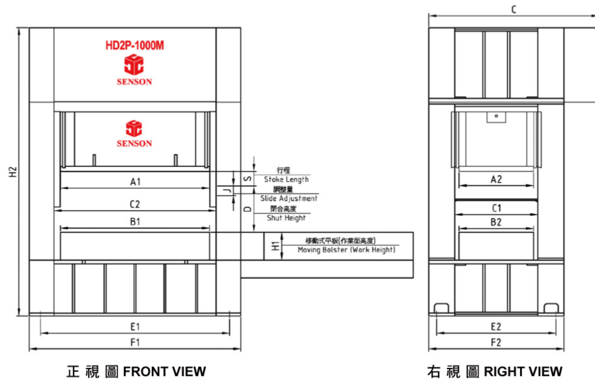
機器外觀尺寸 Major Dimension
