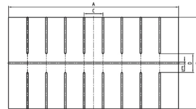
平板尺寸 Bolster Dimension
